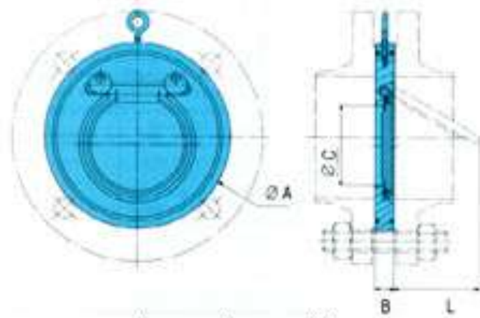
PŘIPOJENÍ MEZI PŘÍRUBY
